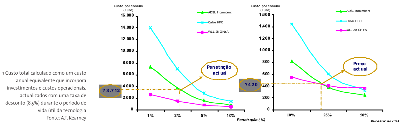
Custo total da tecnologia 1 por conexão vs Penetração (Lisboa e Porto)
