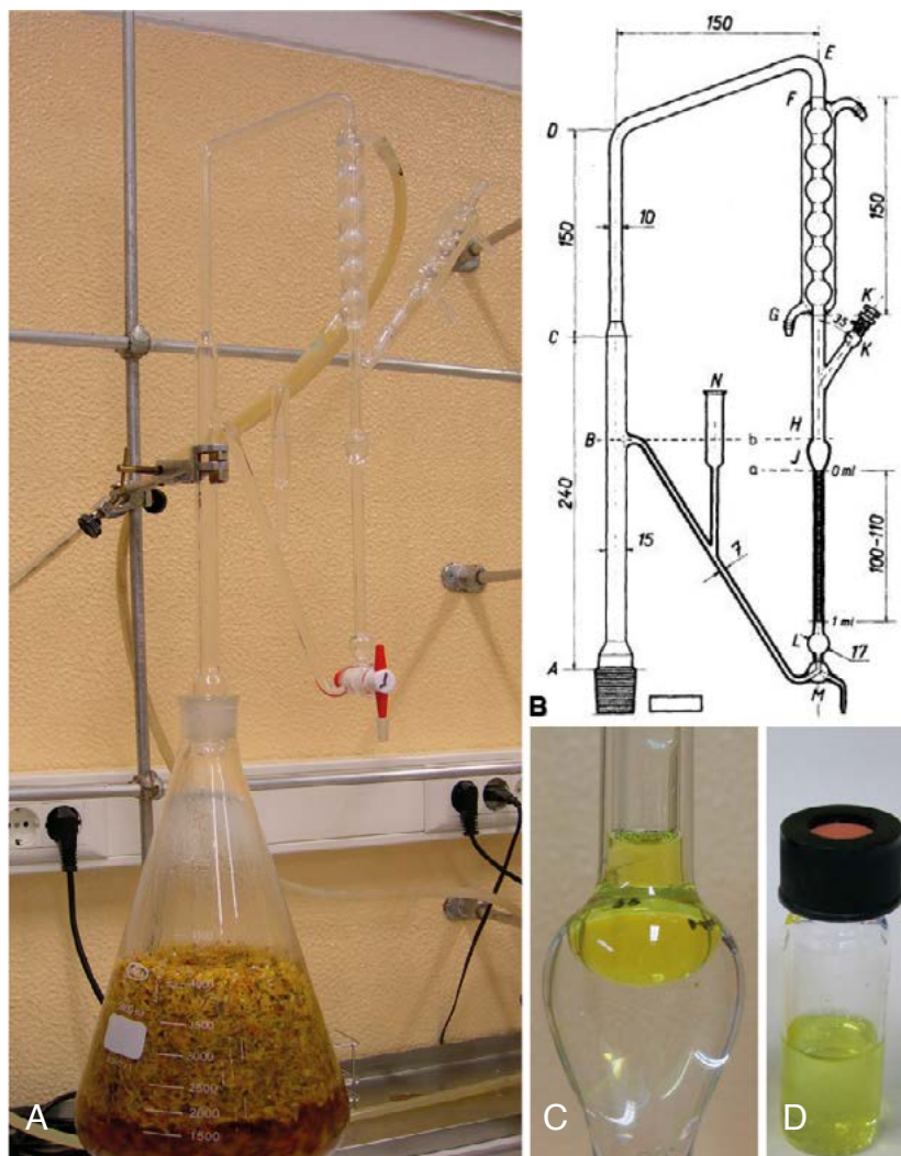
Figura 1 - (A) Aspetto do sistema de hidrodestilação laboratorial, com o aparelho de Clevenger. (B) Esquema do aparelho de Clevenger (adaptado de Lourenço, 2007). (C) Pormenor da ampola de recolha do óleo essencial do aparelho de Clevenger. (D) Pormenor de um frasco de laboratório contendo o óleo essencial.
